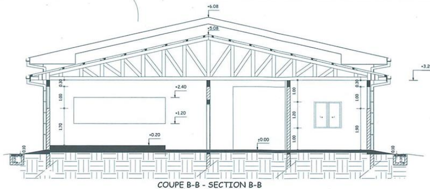
COUPE B-B - SECTION B-B
